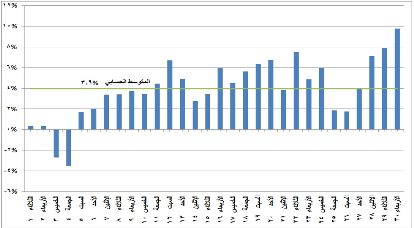
شكل (٩) النسب المئوية للتغير في الحمل الاقصى خلال شهر سبتمبر ٢٠٢٠ مقارنة باليوم المماثل من العام الماضي
