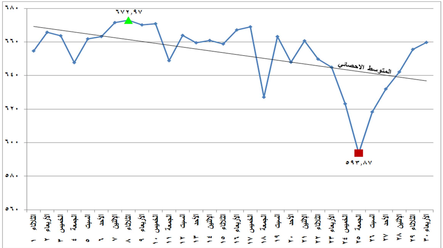
شكل (١٥) إجمالي الطاقة الكهربائية المنتجة من كل المصادر الأولية خلال شهر سبتمبر ٢٠٢٠
