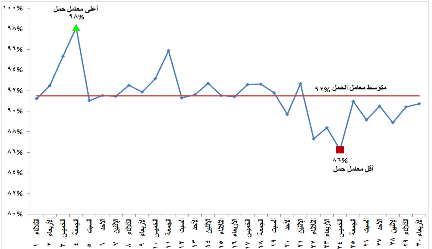
شكل (١٢) إجمالي معامل الحمل لوحدات الانتاج خلال شهر سبتمبر ٢٠٢٠
