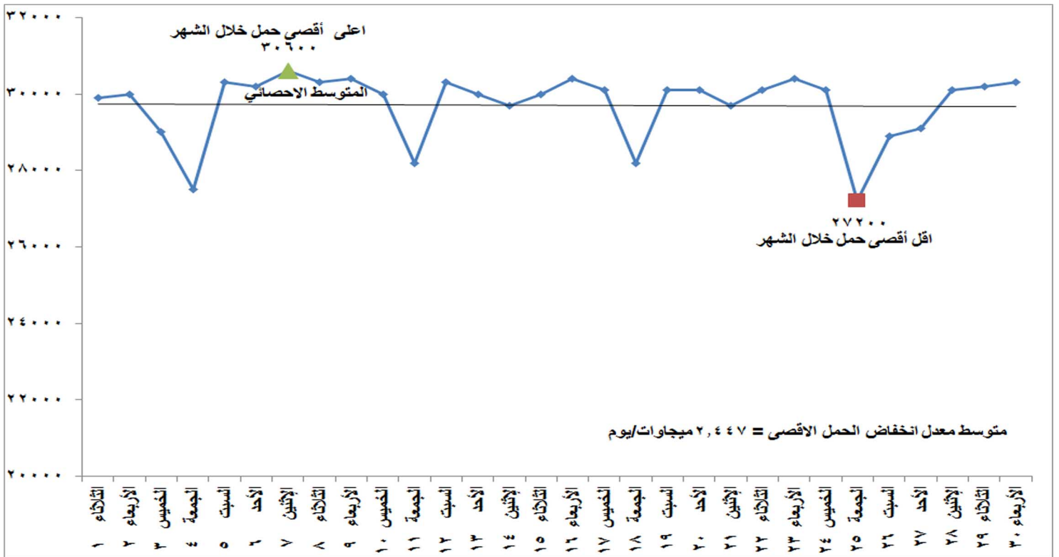
شكل (١) تطور الحمل الاقصى اليومي خلال شهر سبتمبر ٢٠٢٠
