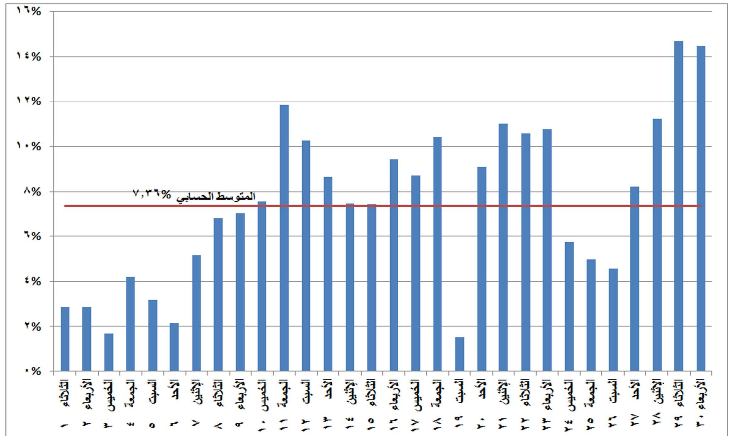
شكل (١٦) نسب التغير في الطاقة الكهربائية المنتجة خلال شهر سبتمبر ٢٠٢٠ مقارنة بالشهر المماثل من العام السابق
