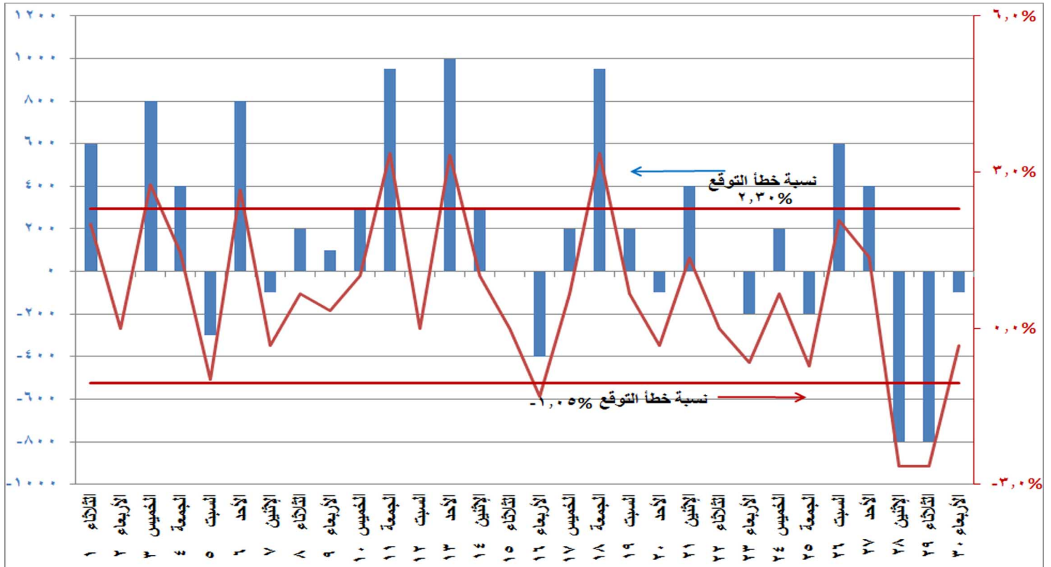
شكل (١٠) الفرق بين الحمل الأقصى المتوقع والمسجل فعليا ونسبة الفرق إلى الحمل المسجل فعليا خلال شهر سبتمبر ٢٠٢٠
