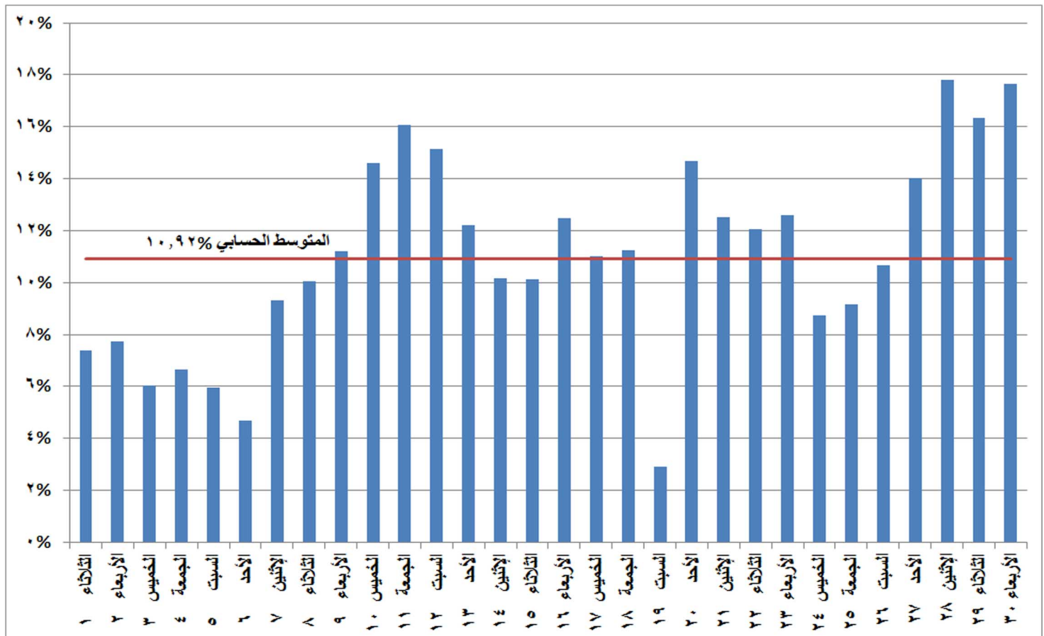
شكل (١٨) نسب التغير في استخدام الغاز الطبيعي في إنتاج الطاقة الكهربائية خلال شهر سبتمبر ٢٠٢٠ مقارنة بالشهر المماثل من العام السابق
