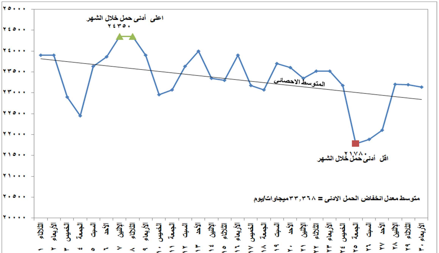
شكل (٢) تطور الحمل الادنى اليومي خلال شهر سبتمبر ٢٠٢٠
