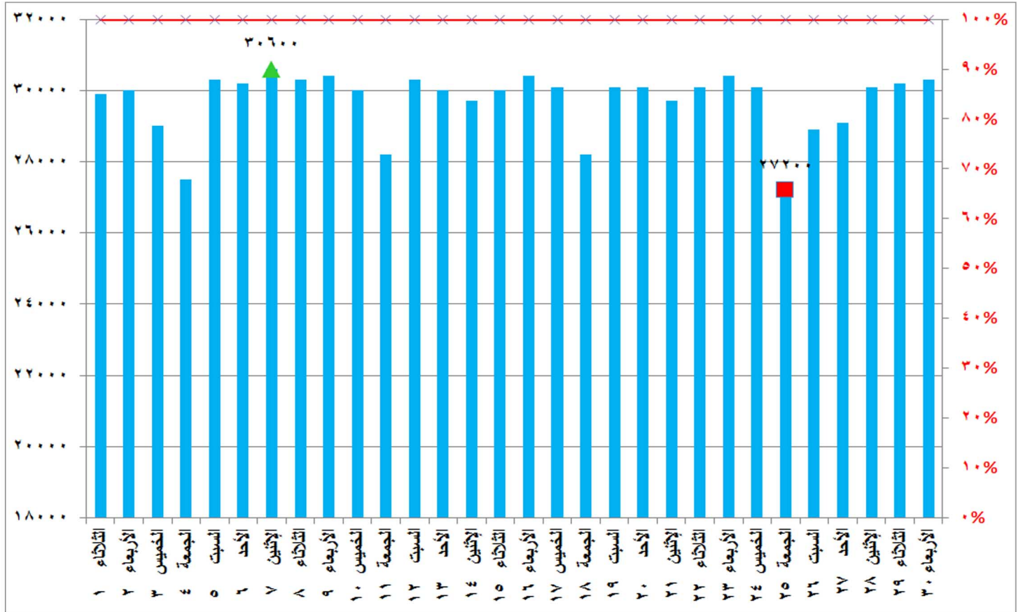
شكل (٥) قدرات الانتاج المتاحة ونسبتها للحمل الأقصى خلال شهر سبتمبر ٢٠٢٠
