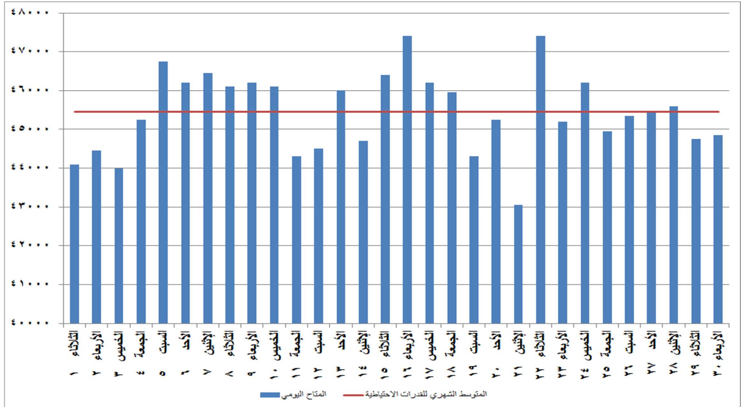
شكل (٢٧) القدرات المتاحة يوميا والمتوسط الشهري للقدرة الاحتياطية خلال شهر سبتمبر ٢٠٢٠
