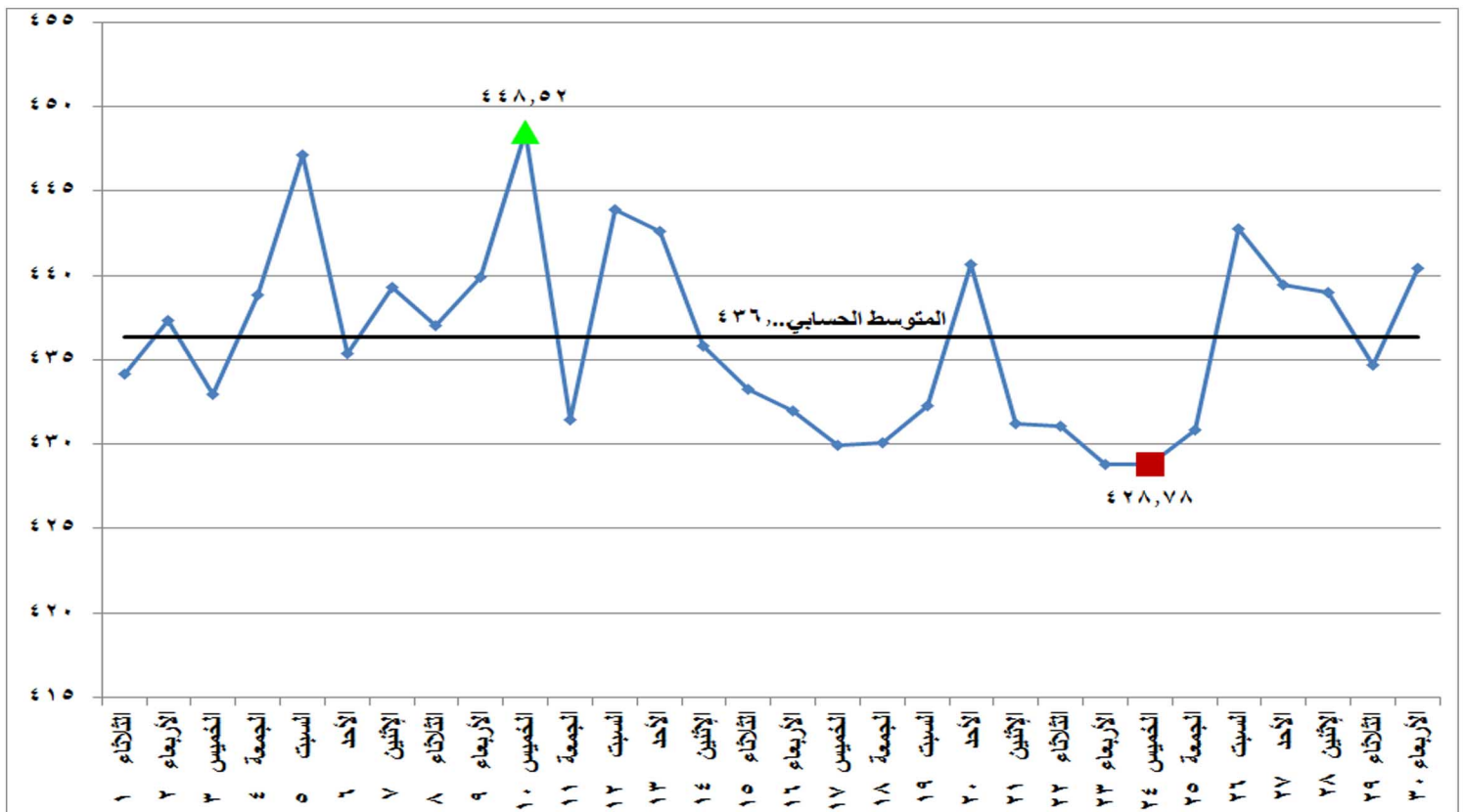
شكل (١٤) معامل انبعاثات غاز ثاني اكسيد الكربون المكافئ على مدى شهر سبتمبر ٢٠٢٠
