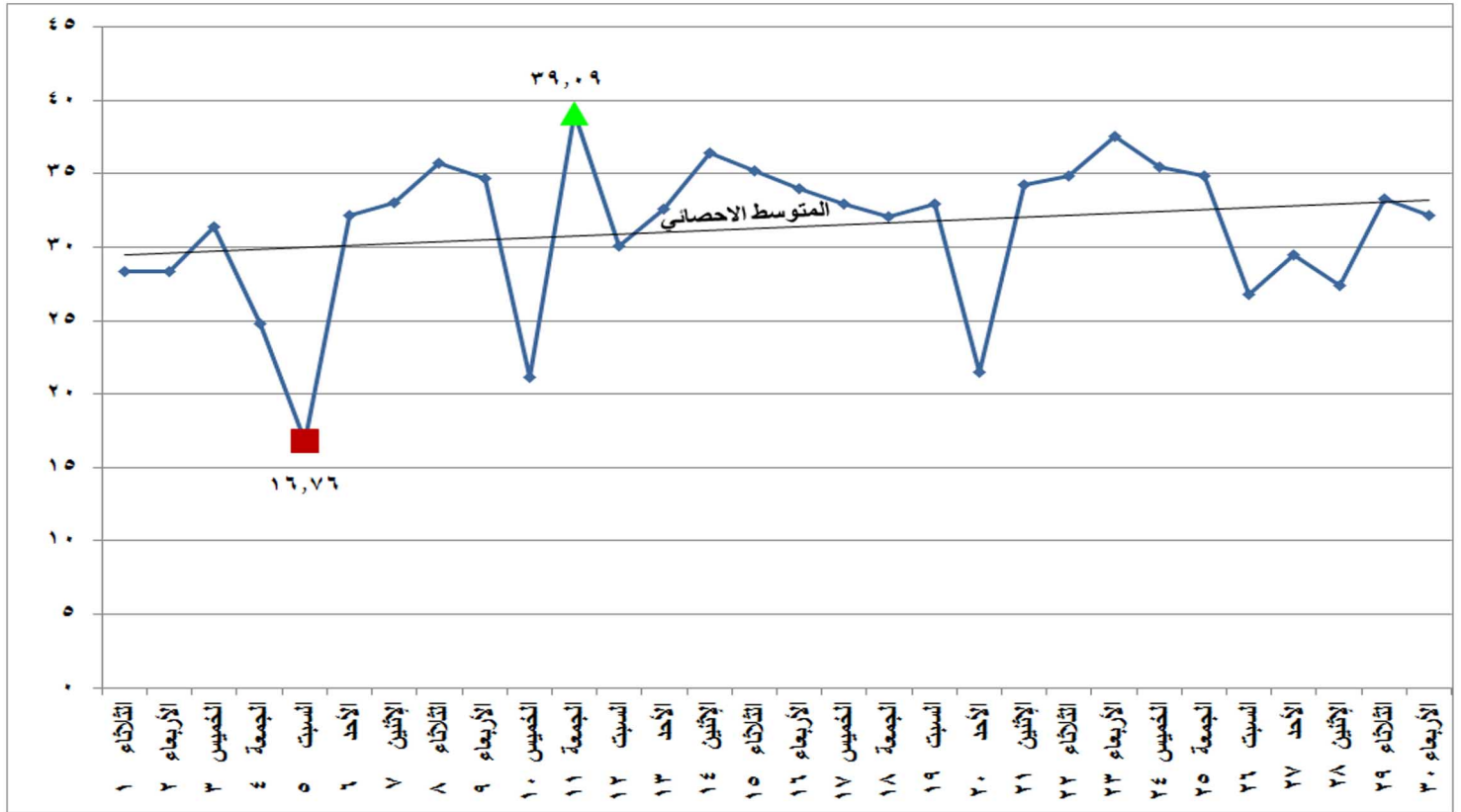
شكل (٢٥) الطاقة الكهربائية المنتجة من الرياح والشمس خلال شهر سبتمبر ٢٠٢٠
