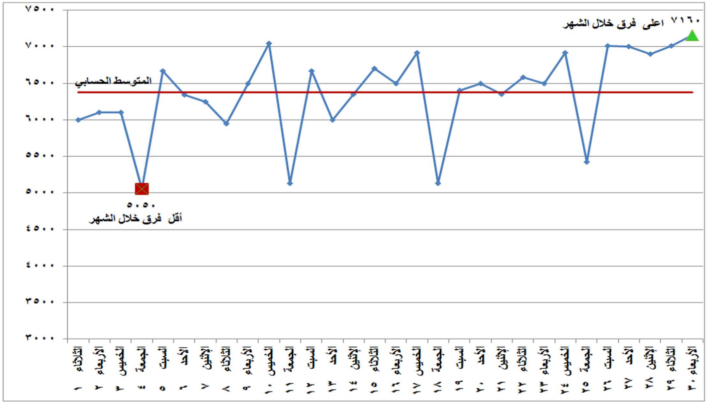
شكل (٣) الفرق بين أقصى وأدنى حمل خلال شهر سبتمبر ٢٠٢٠
