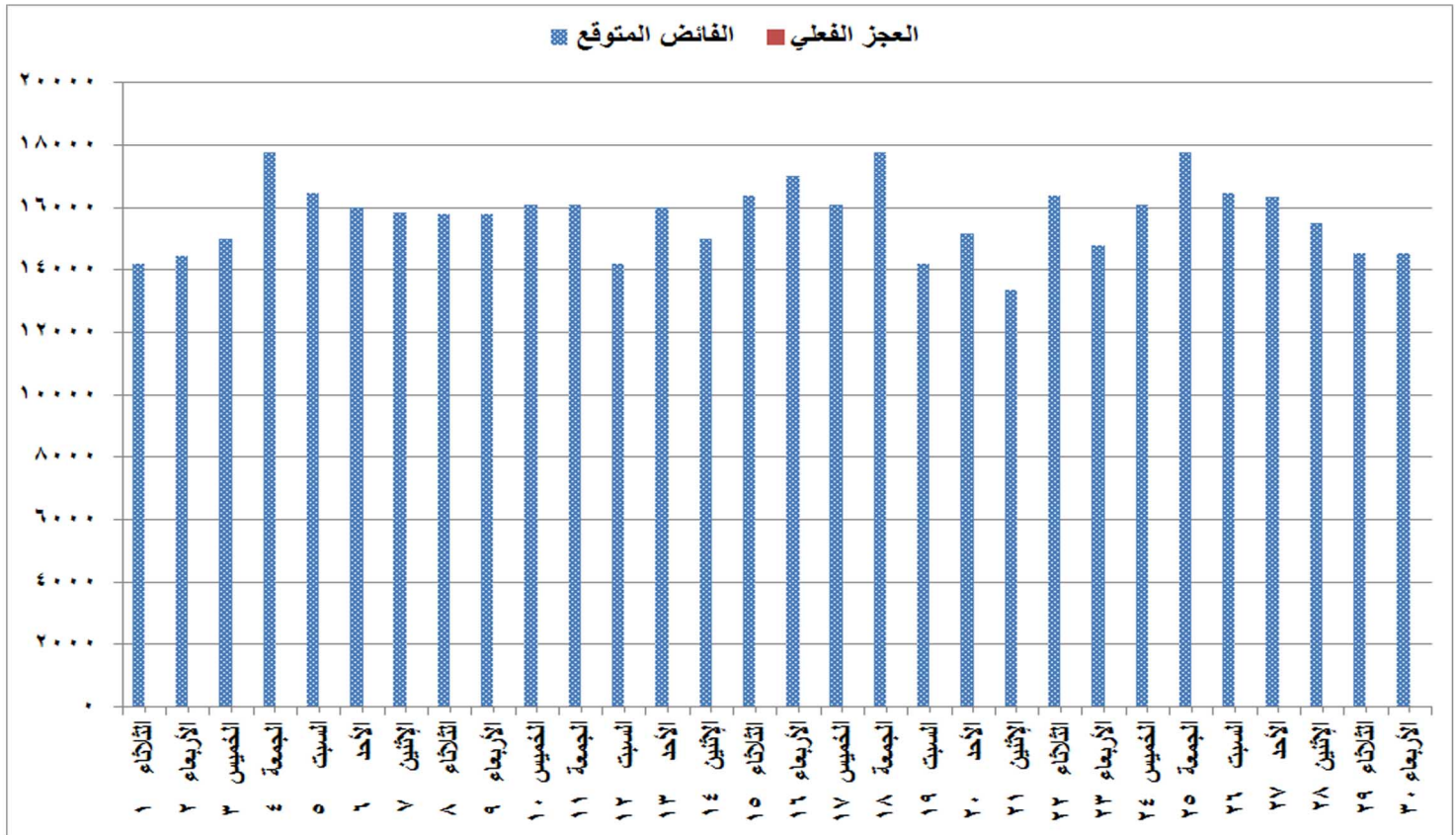
شكل (٧) الفائض والعجز المتوقع للقدرات خلال شهر سبتمبر ٢٠٢٠
