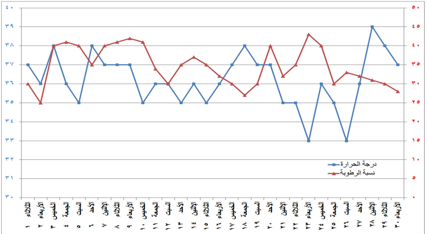
شكل (١١) التغيير في درجة الحرارة والرطوبة النسبية خلال شهر سبتمبر ٢٠٢٠
